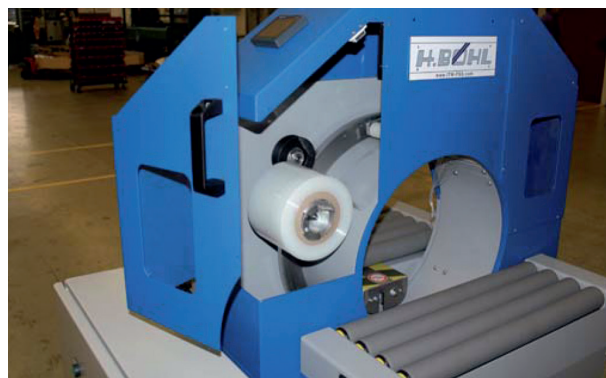
Schnellwechsellvorrichtung für Packmaterialrollen
