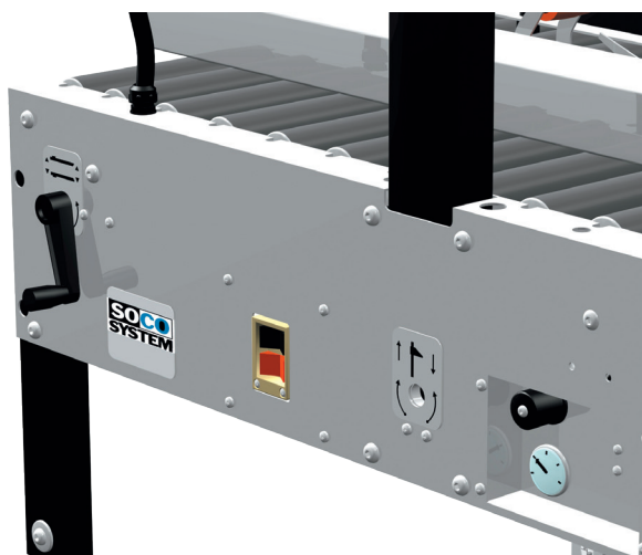
Spindelsystem zur Einstellung von Kartonabmessungen
